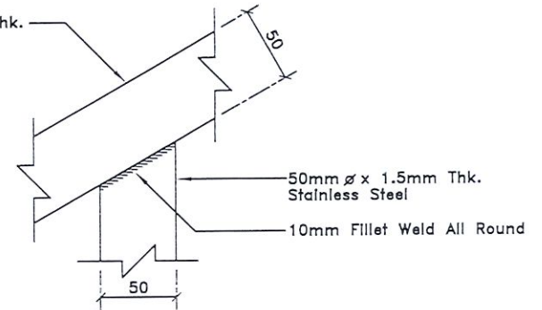
DETAIL 'A' Scale N.T.S
